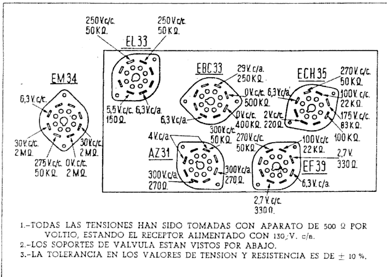
Tensiones y resistencias entre las patillas de las válvulas y mosca
